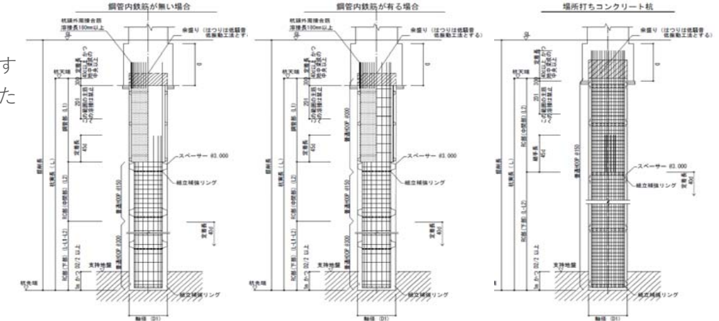
上部鋼管有・鋼管内配筋無し 上部鋼管有・鋼管内配筋有り RC杭(上部鋼管無し)
