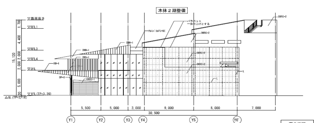
南側立面图
